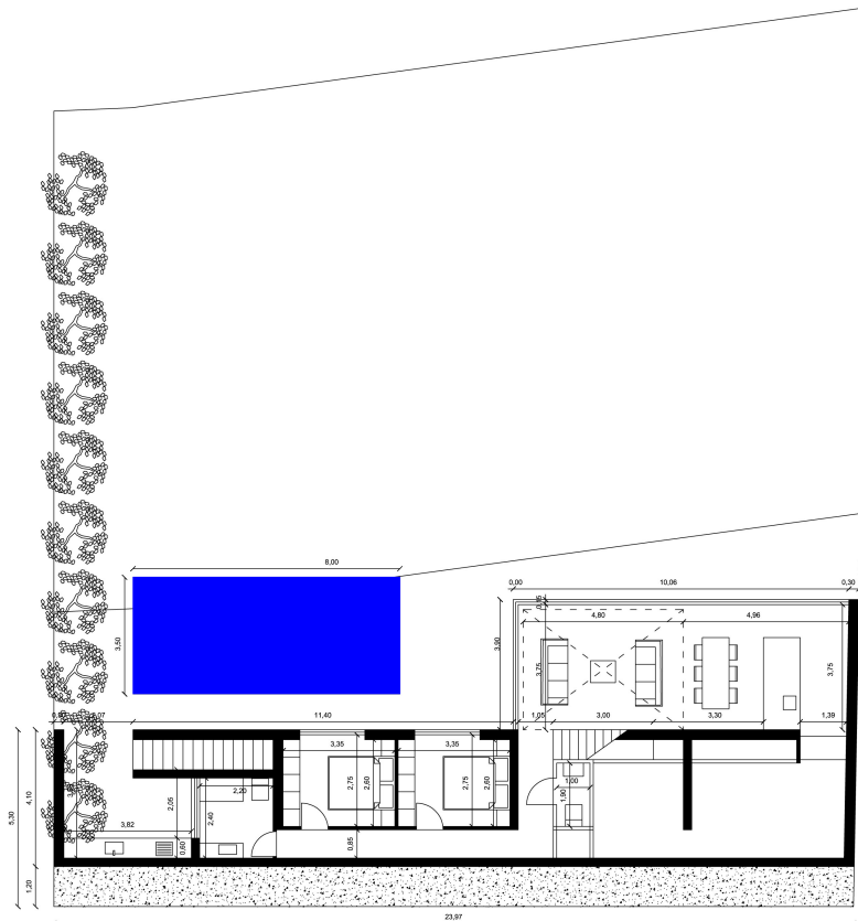
ΚΑΤΩΦΗ ΙΣΟΓΕΙΟΥ
